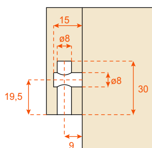
Găurirea pentru laterale 18 mm
