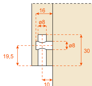
Găurirea pentru laterale 19/20 mm
